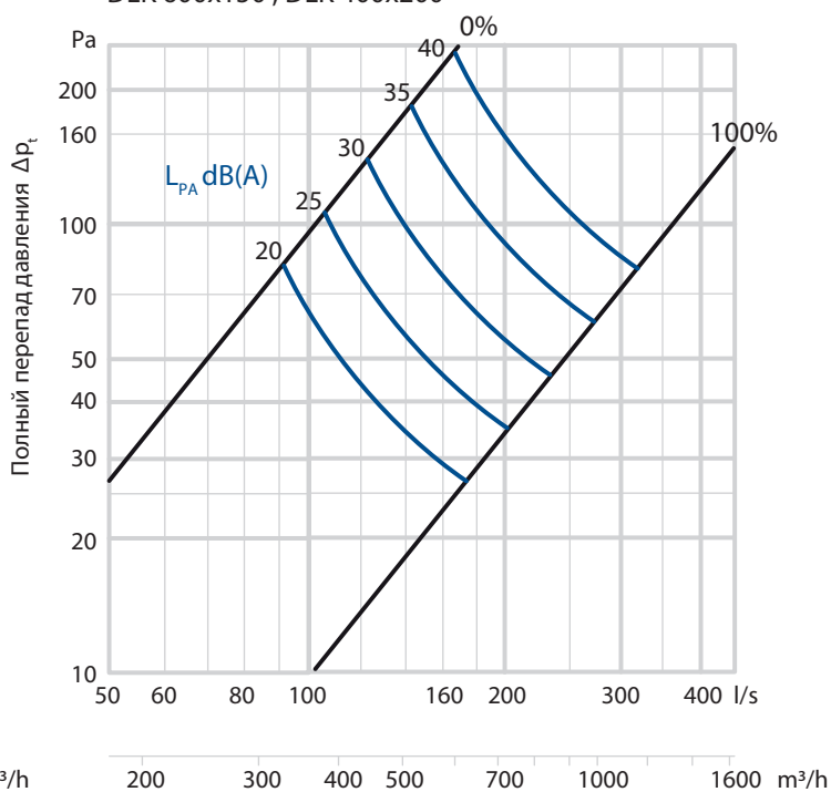
D.8. DLK 600x150 ; DLK 400x200
