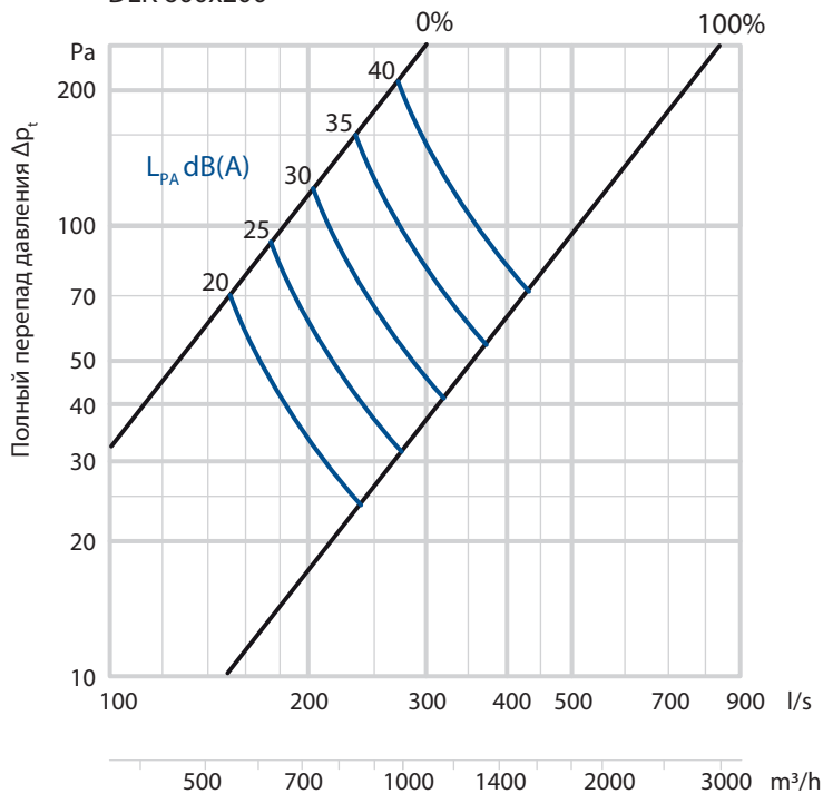
D.10. DLK 600x200
