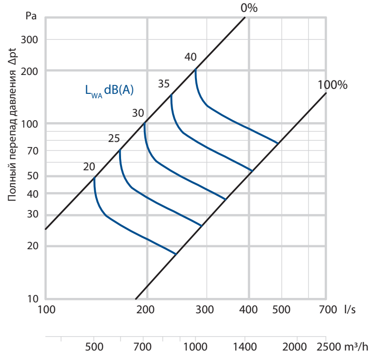
D.6. ТК 400-315
