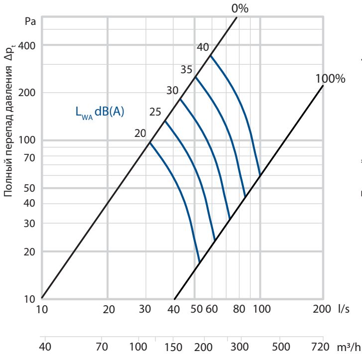
D.3. TK 200-160
