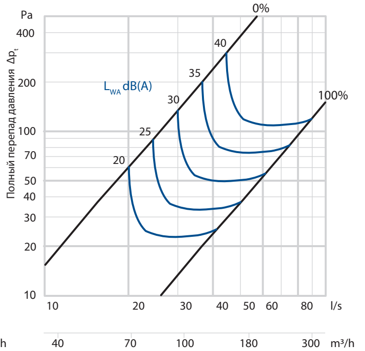
D.2. TK 160-125
