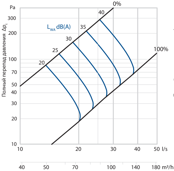
D.1. TK 125-100
